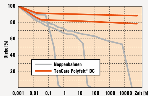
Dickenreduktion bei 200 kPa Auflast über einen längeren Zeitraum. (Prüflabor: GEOTRAC/UK)
